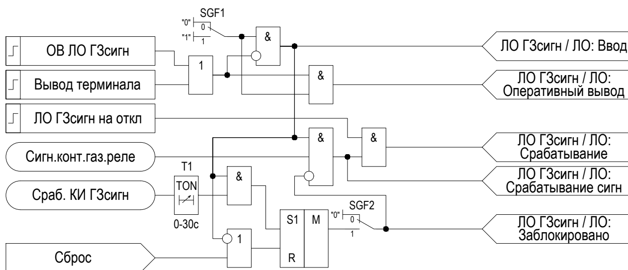
Рисунок 2.19 – Функциональная схема «ЛО ГЗсигн»
