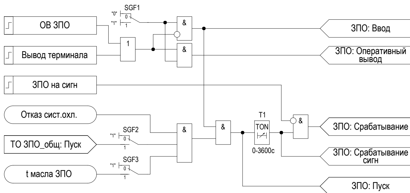
Рисунок 2.12 – Функциональная схема «ЗПО»
