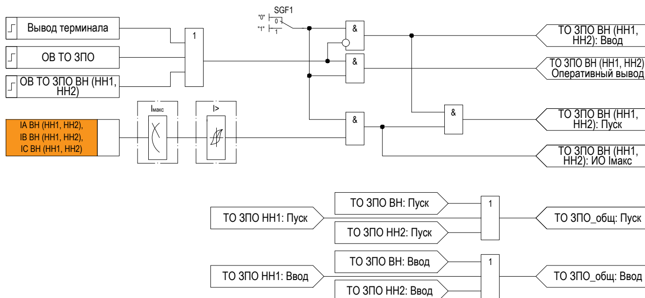
Рисунок 2.13 – Функциональная схема «ТО ЗПО»
