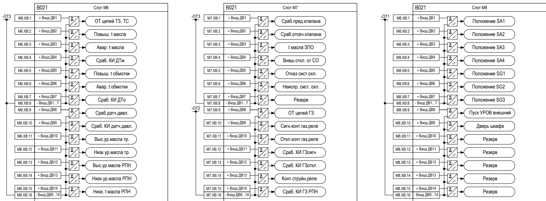
Рисунок Г.3 – Подключение дискретных входов и выходов к внутренним сигналам алгоритмов для плат в слотах M6-M8
