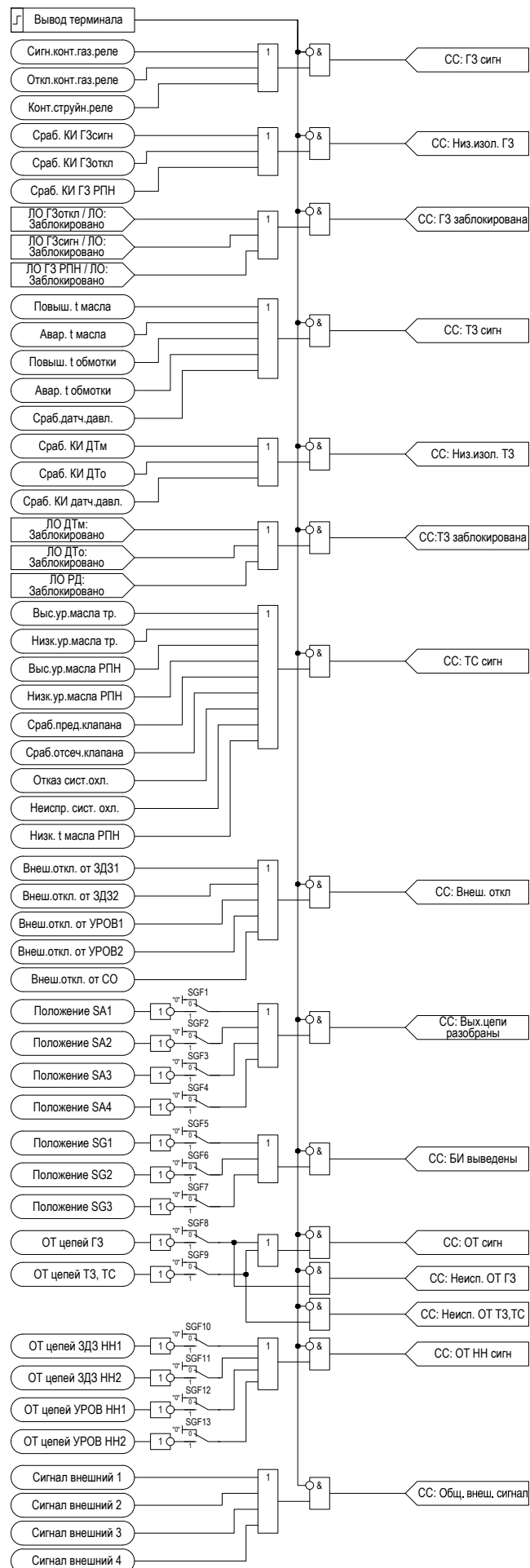
Рисунок 2.33 – Функциональная схема «СС»
