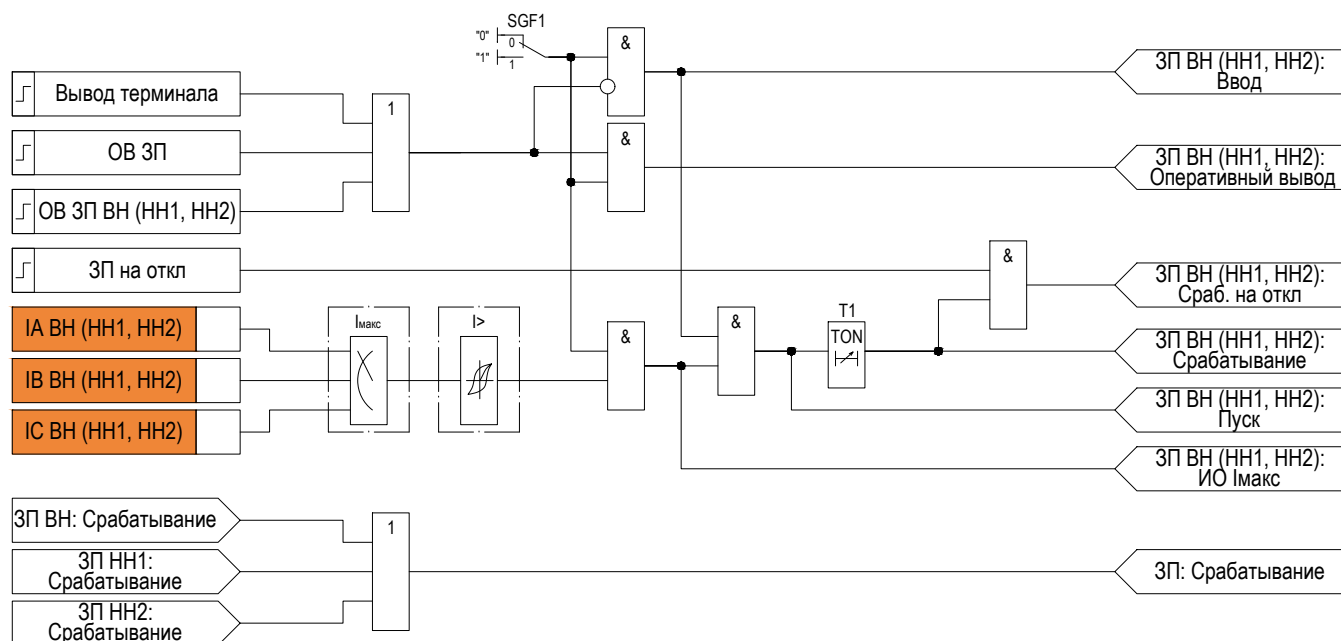
Рисунок 2.14 – Функциональная схема «ЗП»
