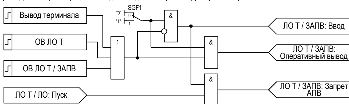
Рисунок 2.28 – Функциональная схема «ЗАПВ»
