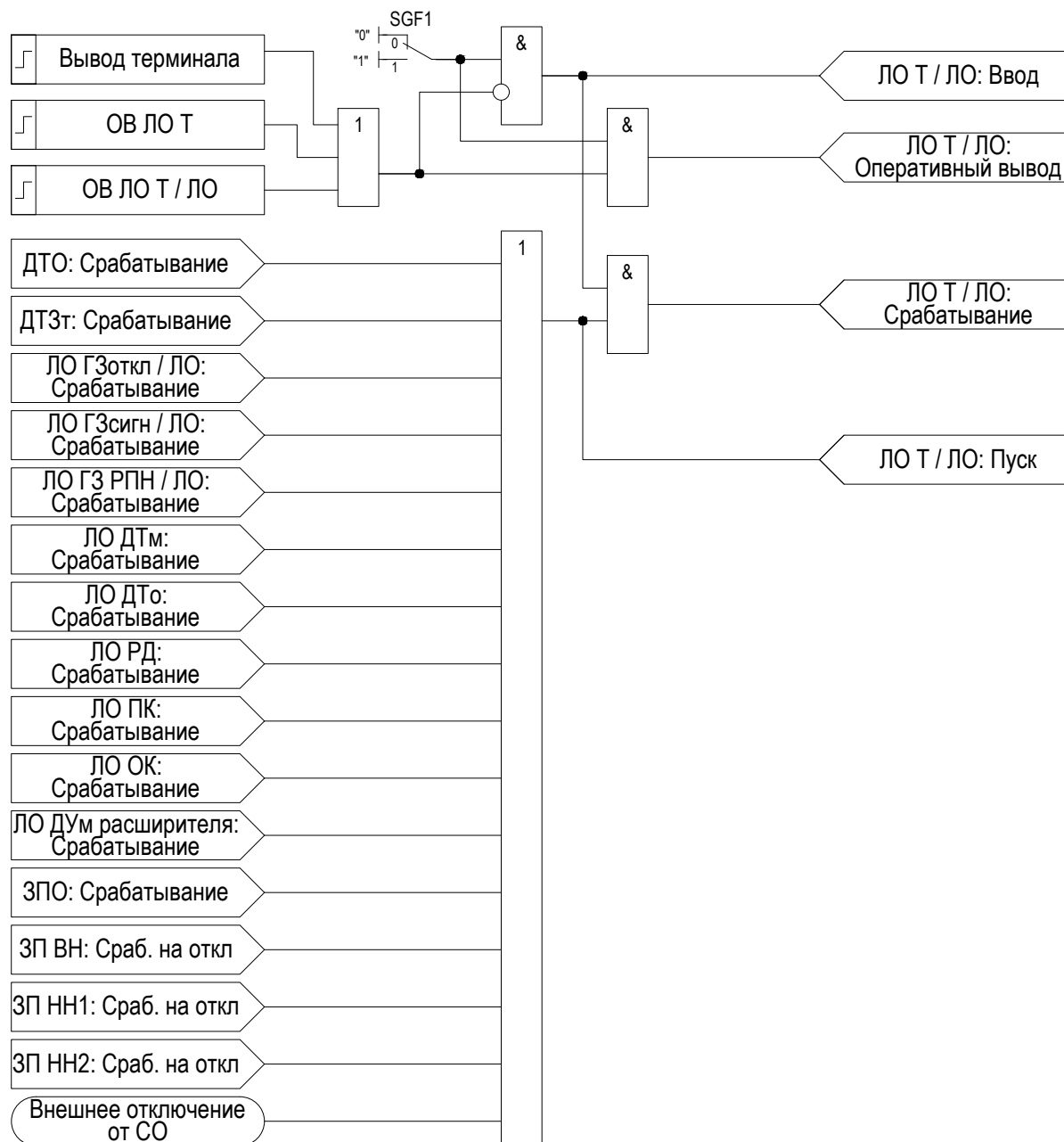
Рисунок 2.27 – Функциональная схема «ЛО»
