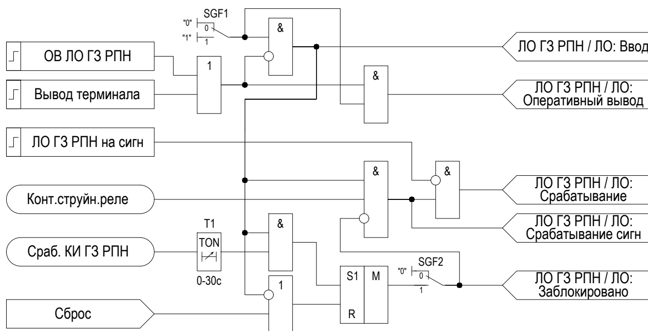
Рисунок 2.20 – Функциональная схема «ЛО ГЗ РПН»
