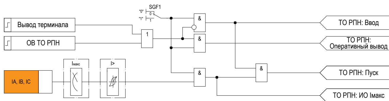
Рисунок 2.17 – Функциональная схема «ТО РПН»
