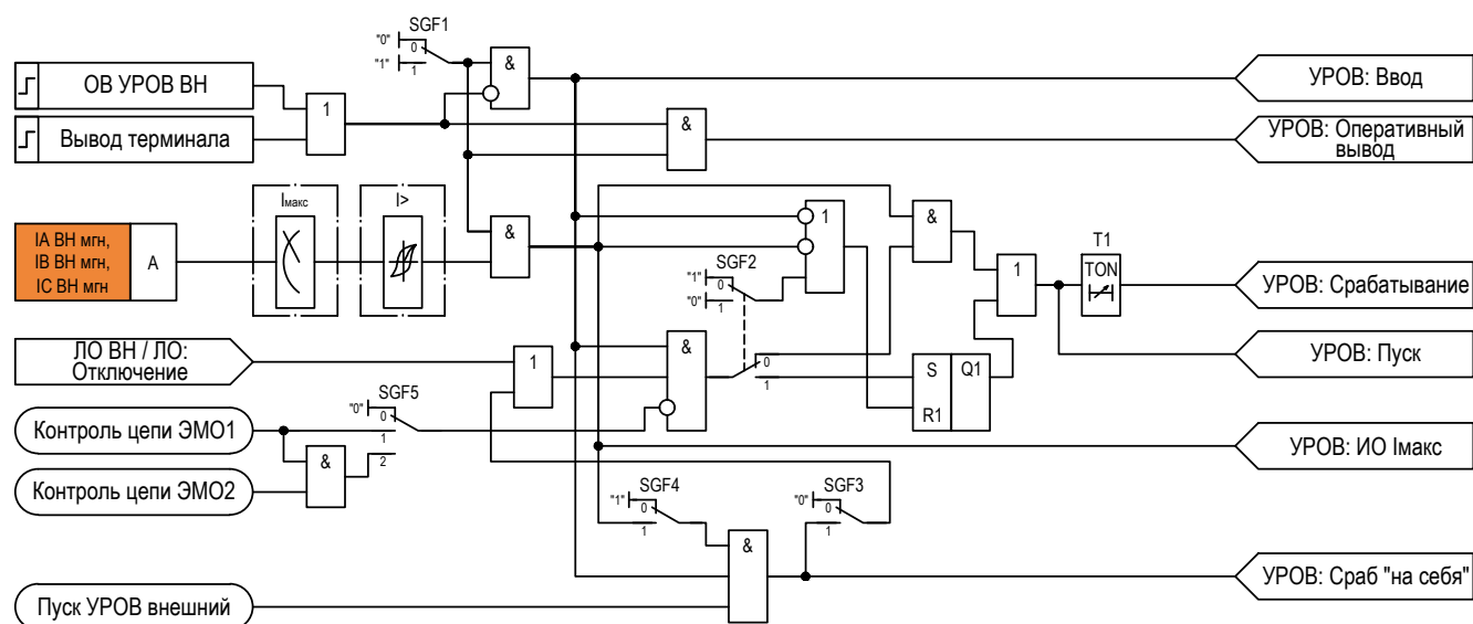
Рисунок 2.32 – Функциональная схема «УРОВ»
