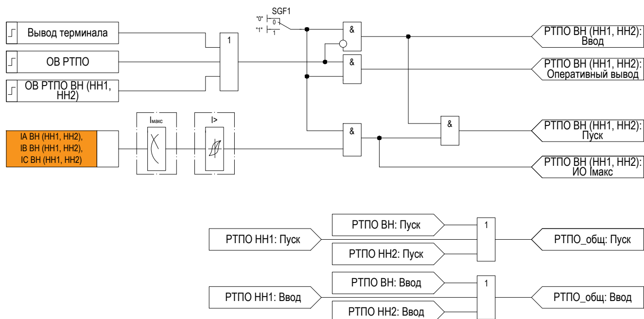
Рисунок 2.15 – Функциональная схема «РТПО»
