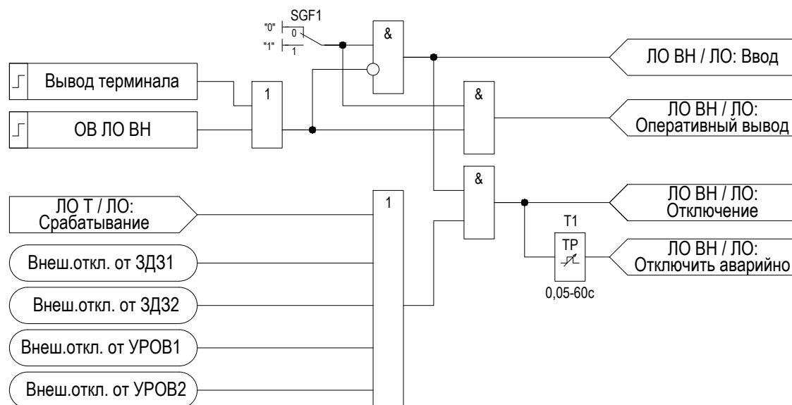
Рисунок 2.29 – Функциональная схема «ЛО»
