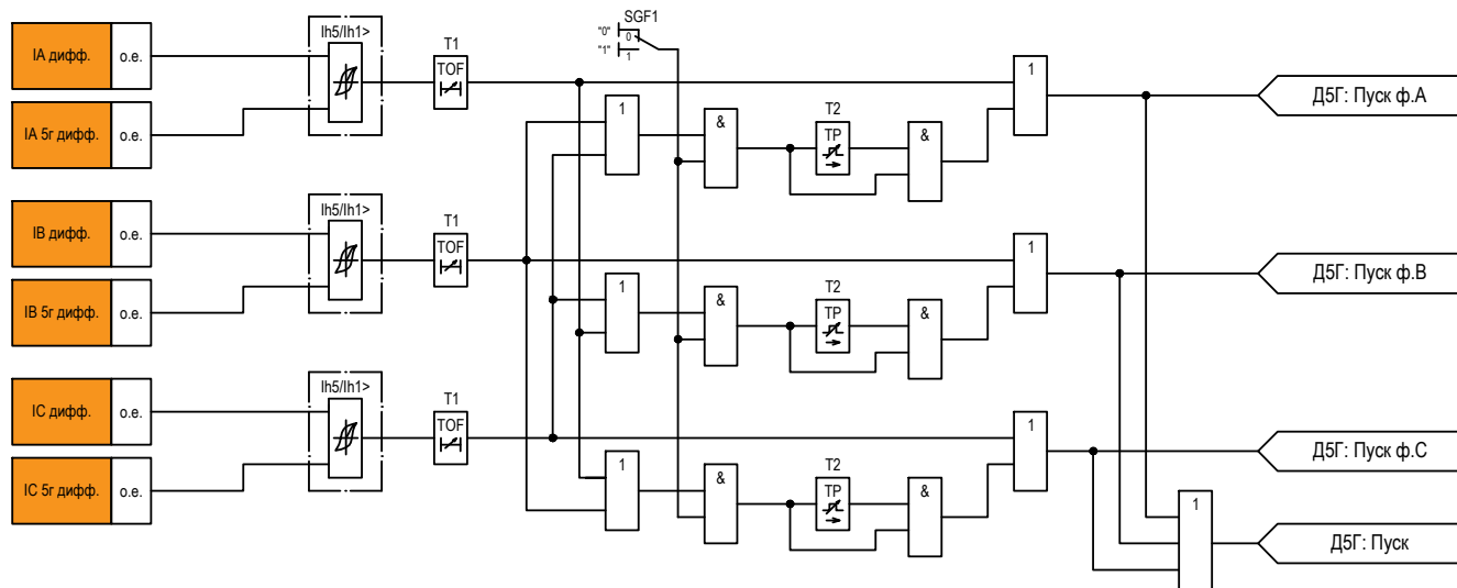
Рисунок 2.6 – Функциональная схема «Д5Г»
