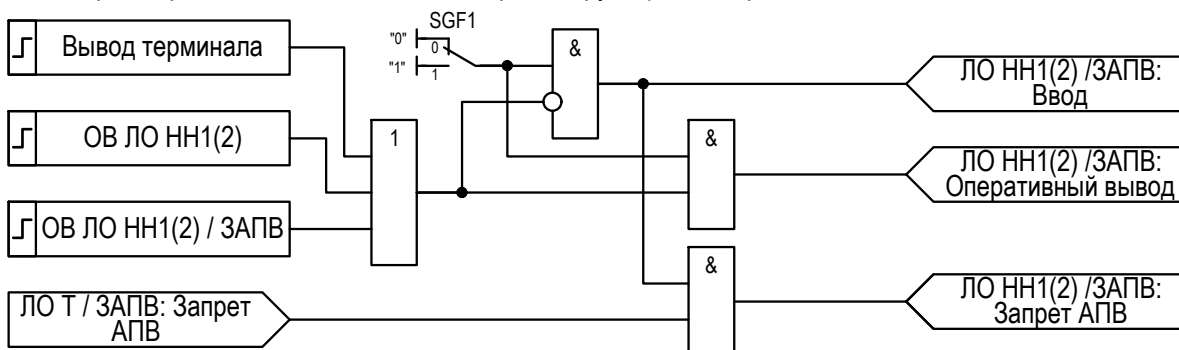
Рисунок 2.31 – Функциональная схема «Запрет АПВ»
