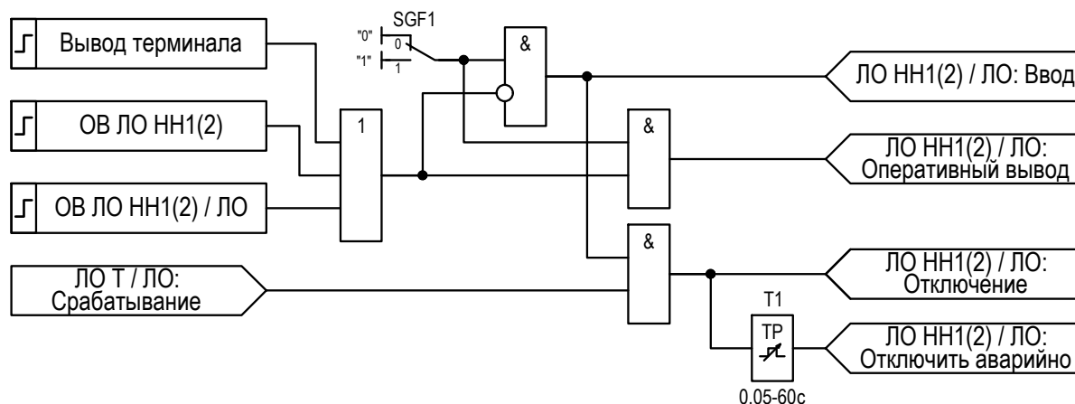
Рисунок 2.30 – Функциональная схема «ЛО»
