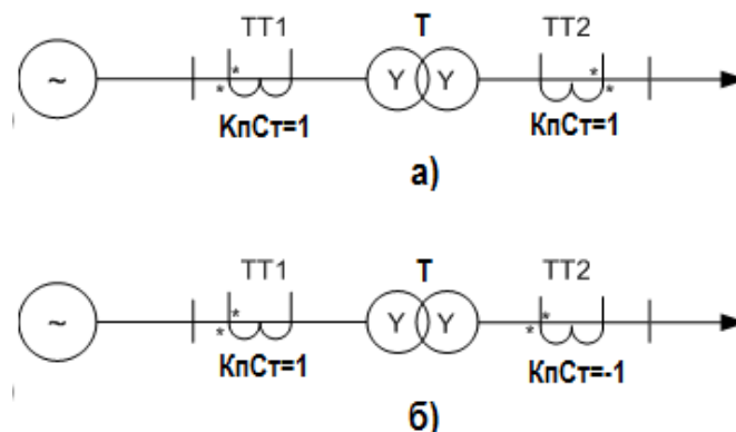
Рисунок 2.1 – Поясняющая схема включения трансформаторов тока: (а) противофазное включение ТТ (б) синфазное включение ТТ
